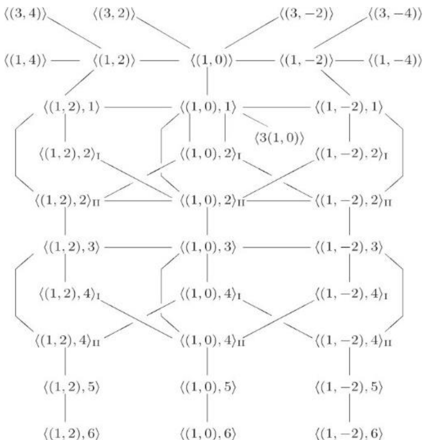
Рис. 1. Комплексные схемы неособых кривых бистепени (4,3) на гиперboloиде
