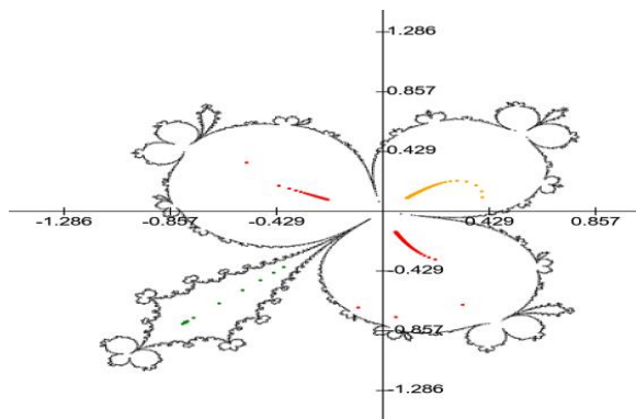
Рис.3. Три лепестка Ло Фату и притягивающая неподвижная точка функции f_{(1+i)\cos(0,65)}(z) = z^5 + (1 + i)\cos(0,65)z^4 + z
