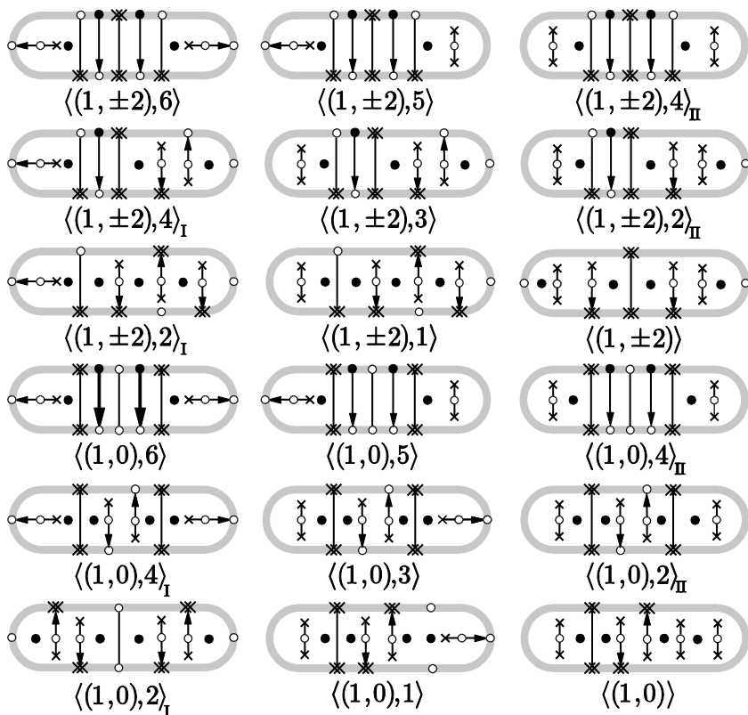
Рис. 3. Канонические скелеты негиперболических кривых
