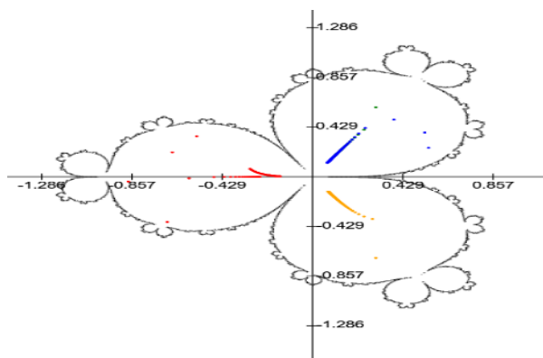
Рис.1. Три лепестка Ло-Фату функции f_0(z) = z^4 + z
