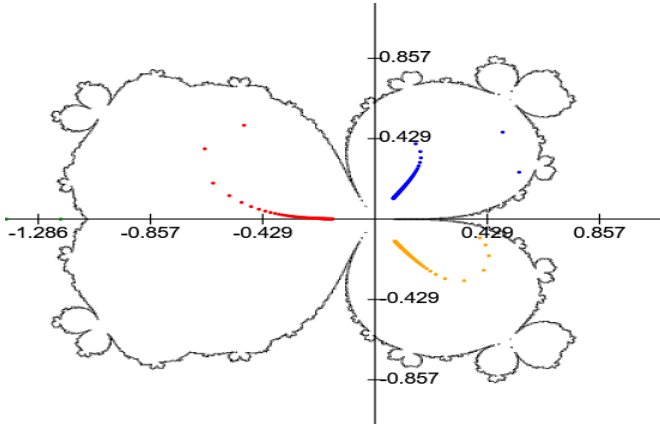
Рис. 2. Три лепестка Ло-Фату и отталкивающая неподвижная точка функции f_{1,1}(z) = z^5 + 1,1z^4 + z
