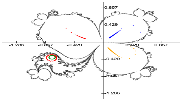
Рис. 4. Три лепестка Ло-Фату и диск Зигеля функции f_{0,753+i0,369}(z) = z^5 + (0,753 + i0,369)z^4 + z
