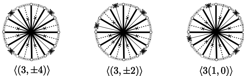
Рис. 2. Канонические графы гиперболических кривых
